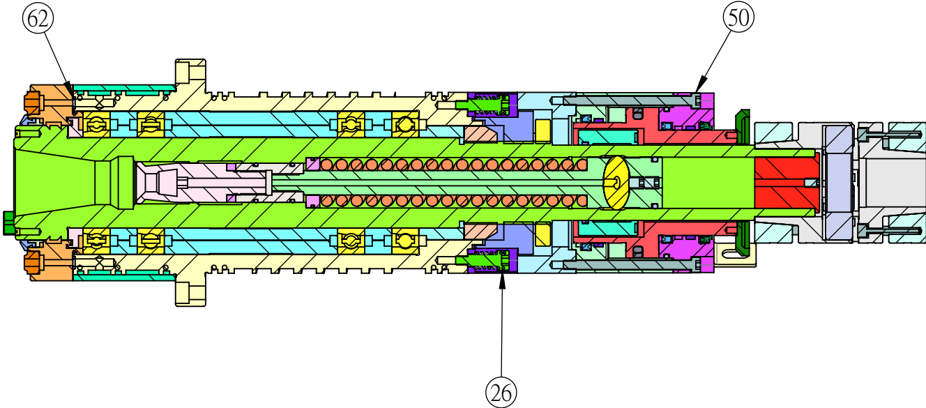
剖面圖 B-B 比例 1 : 3.5
