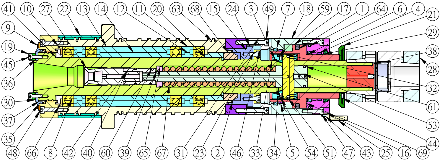
剖面圖 A-A 比例 1 : 3.5
